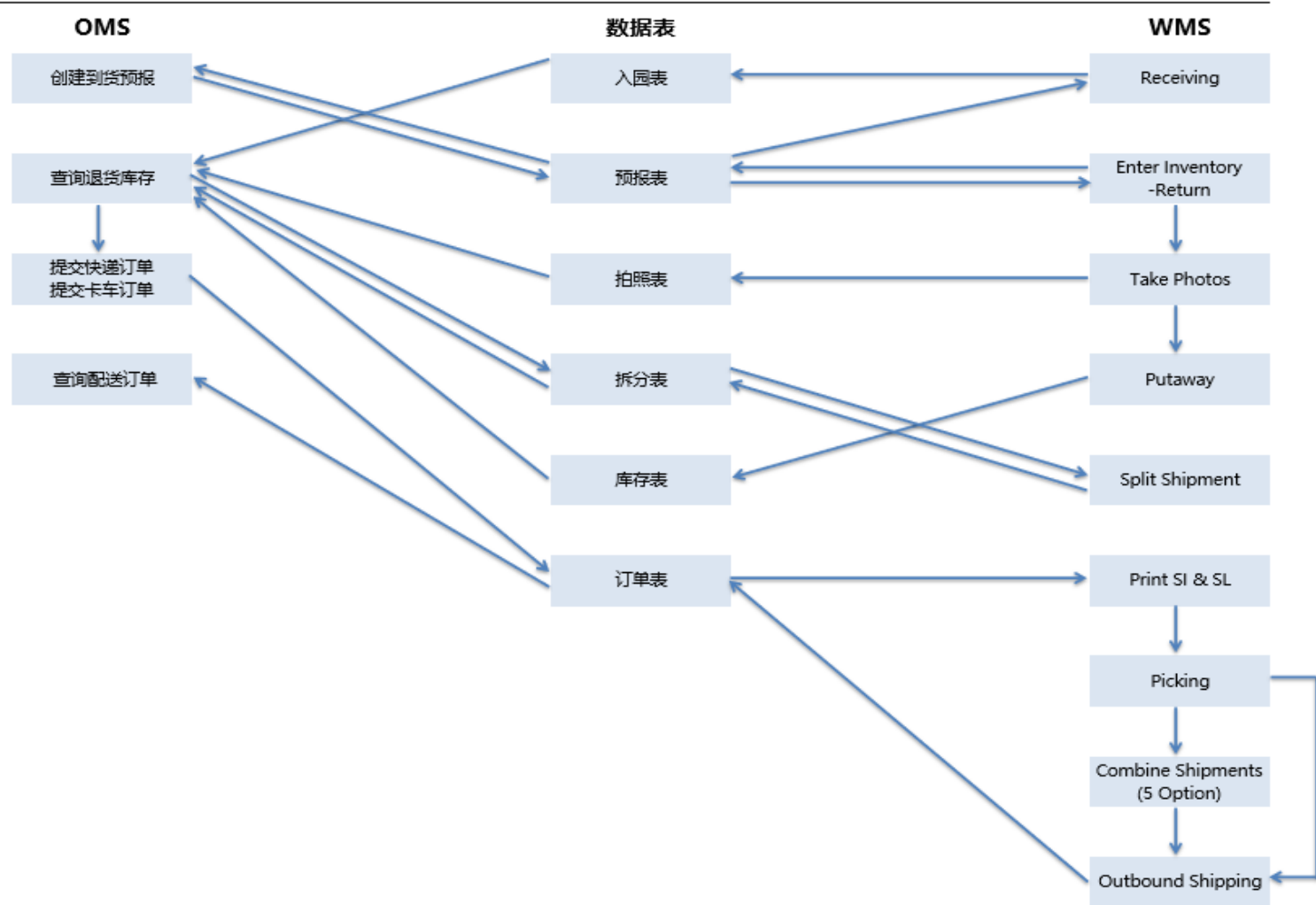
退货处理总体流程图
